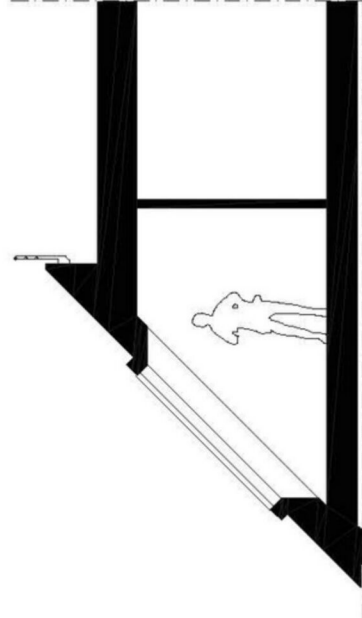
SCHNITT B
