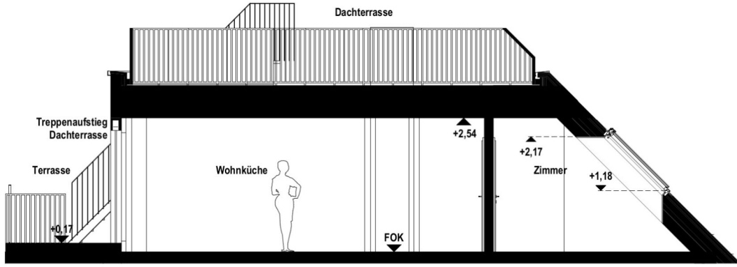
Schnitt
