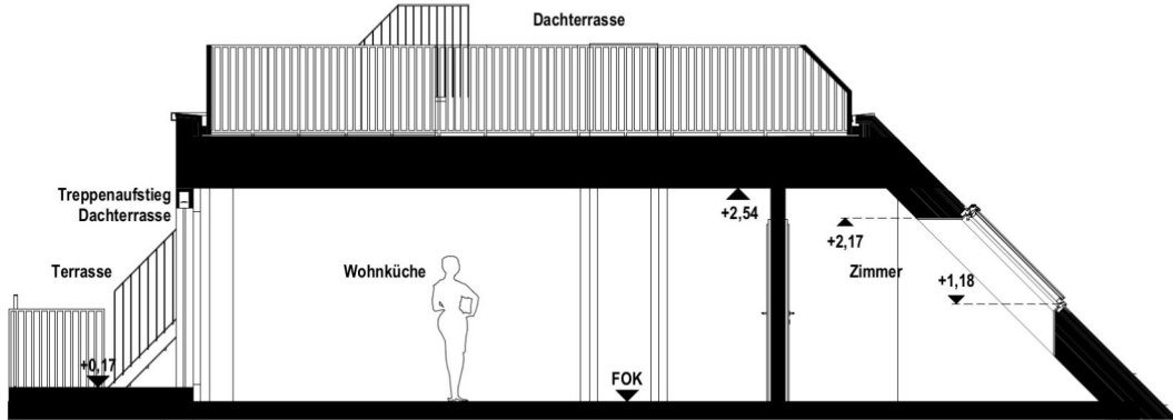
Schnitt
