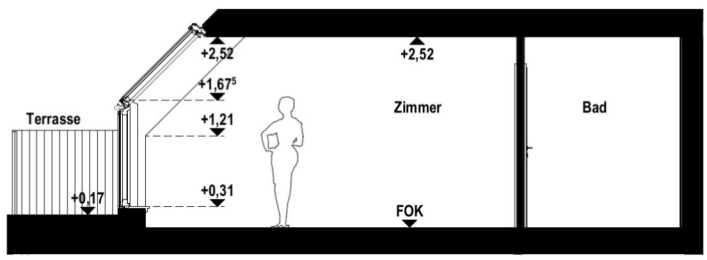
Schnitt
