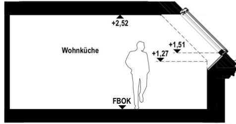
Schnitt
