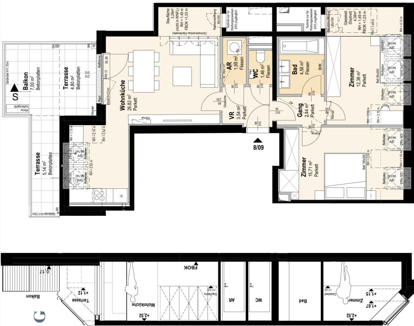
Schnitt
