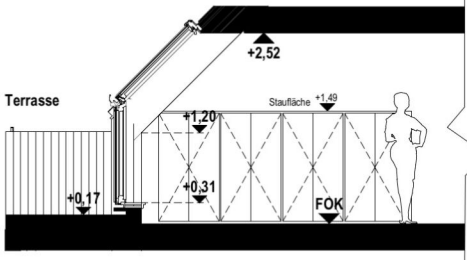
Schnitt 2
