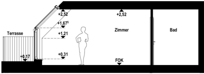
Schnitt
