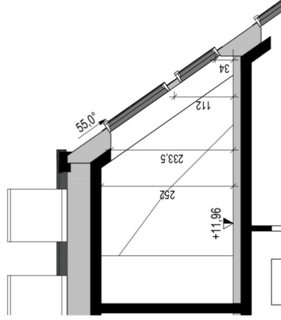
Schnitt 20.B
