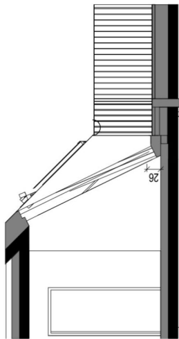
Schnitt 44.B
