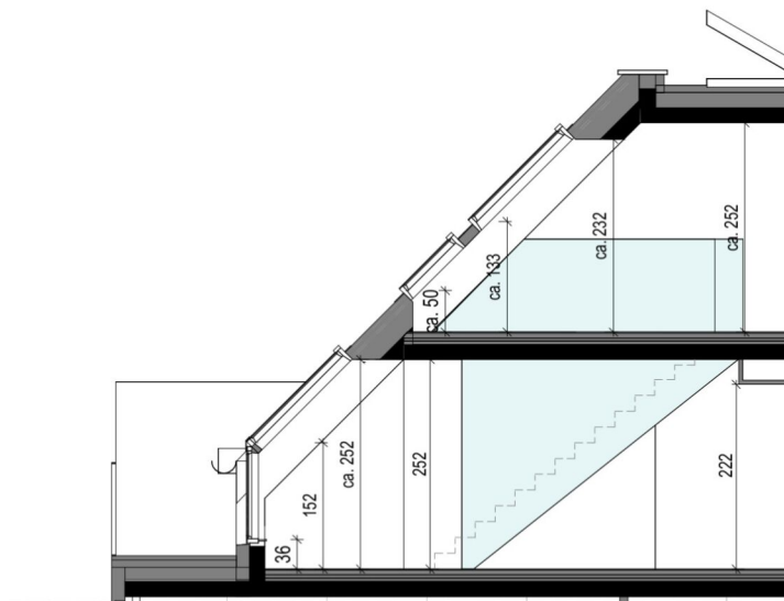
Schnitt 48.B
