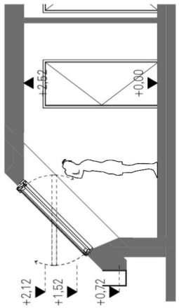
Schnitt 1
