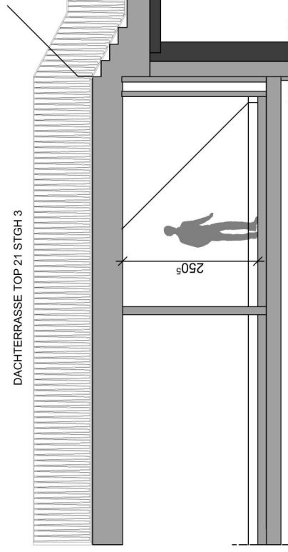
SCHNITT 3-3
