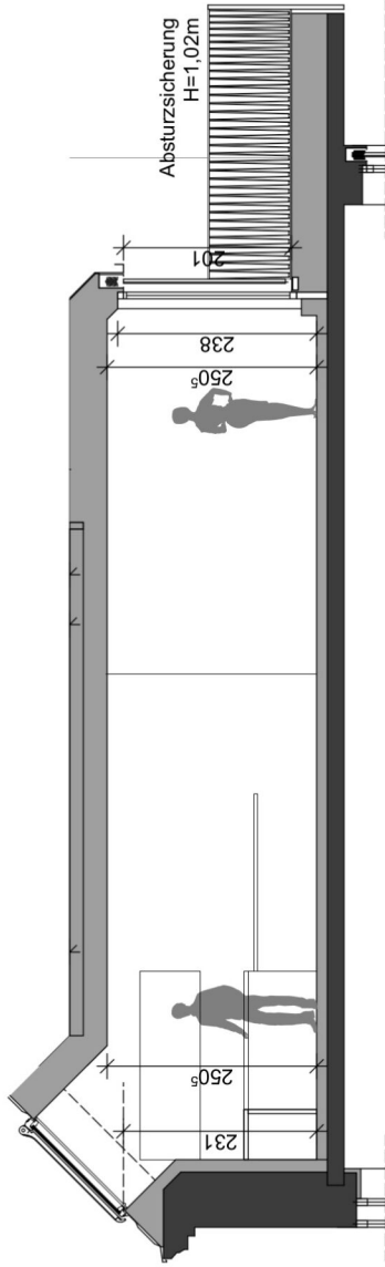
SCHNITT 1-1
