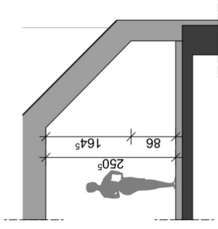
SCHNITT 2-2
