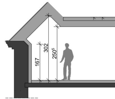
SCHNITT 4-4
