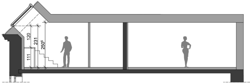
SCHNITT 3-3
