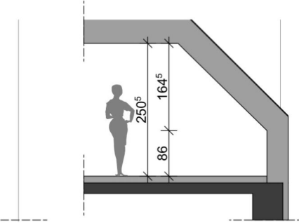
SCHNITT 2-2
