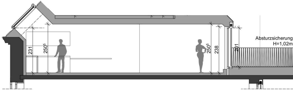
SCHNITT 1-1
