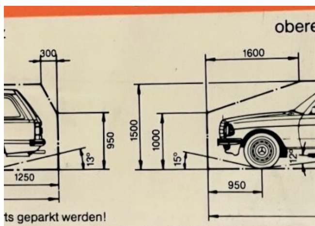
Abmessungen Garage
