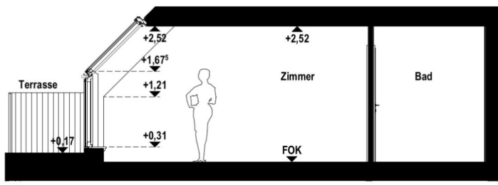
Schnitt
