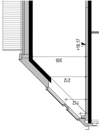
Schnitt 31.A
