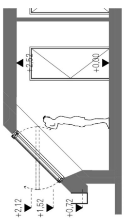
Schnitt 1
