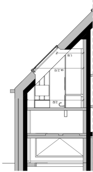
Schnitt 51.A M 1:100
