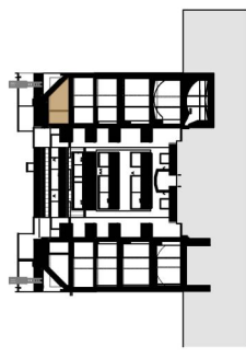
SCHNITT 3-3
