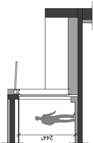
SCHNITT 3-3
