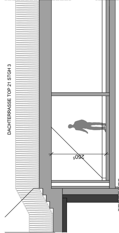
SNITT 3-3
