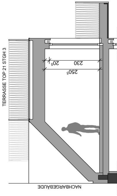
SNITT 1-1
