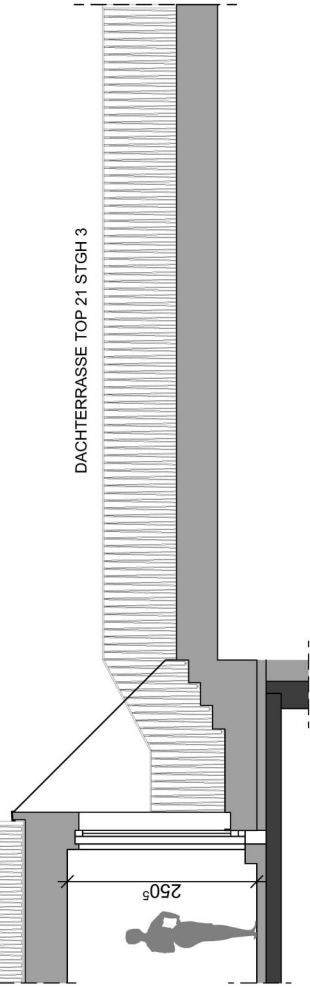
SCHNITT 2-2
