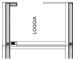
SCHNITT A-A
