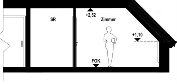
Schnitt
