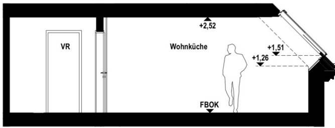
Schnitt
