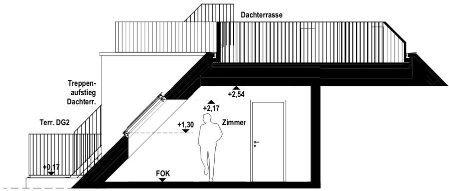
Schnitt
