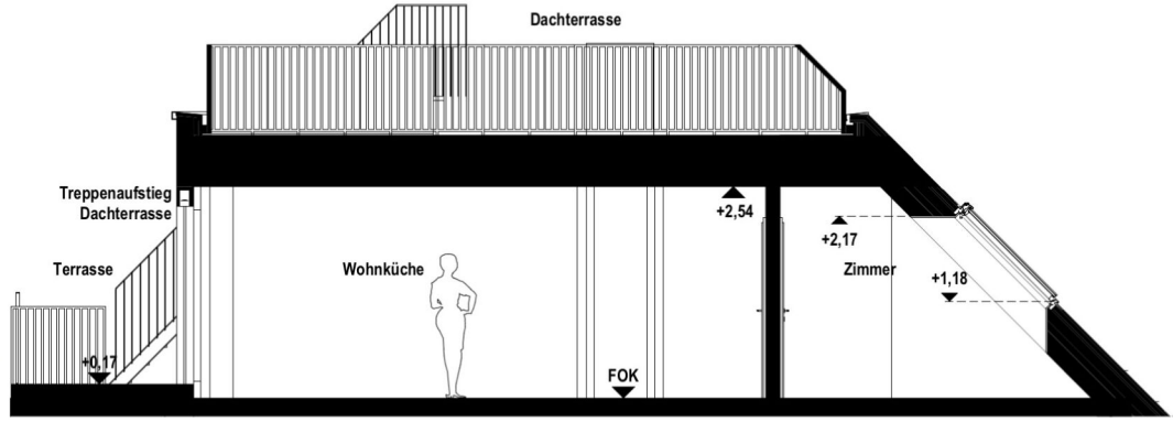
Schnitt
