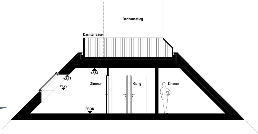
Schnitt
