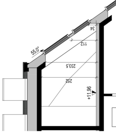
Schnitt 20.B
