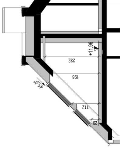
Schnitt 20.A
