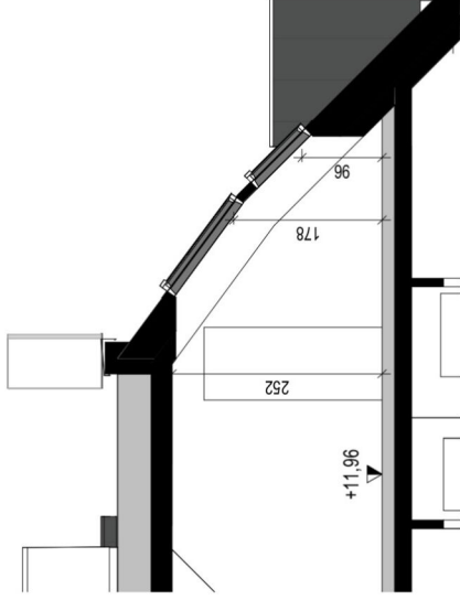
Schnitt 20.C
