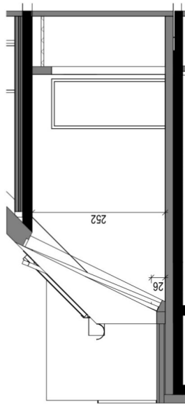
Schnitt 49.B
