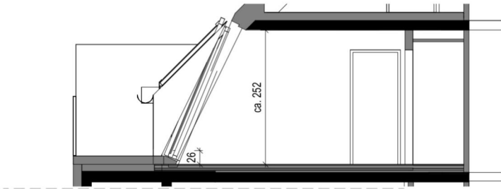
Schnitt 48.A
