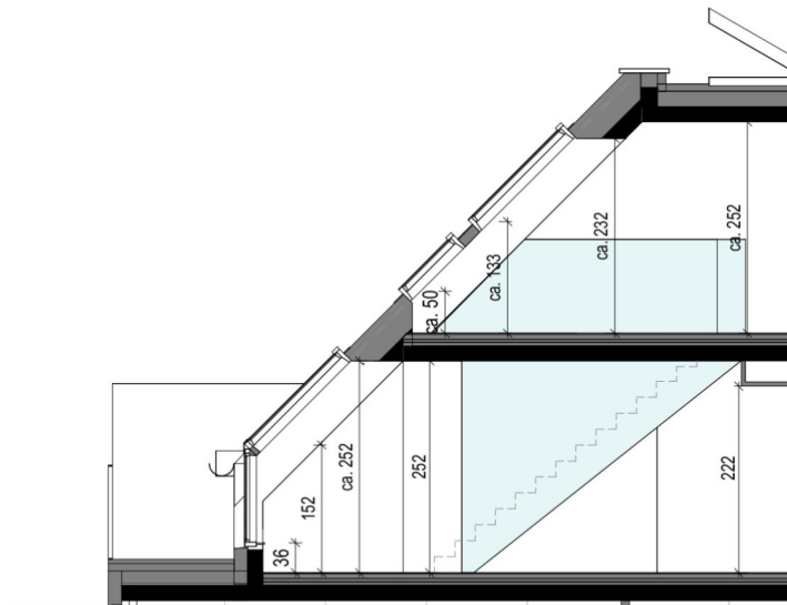
Schnitt 48.B
