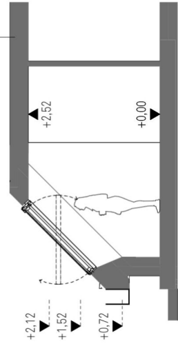
Schnitt 1
