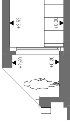
Schnitt 2
