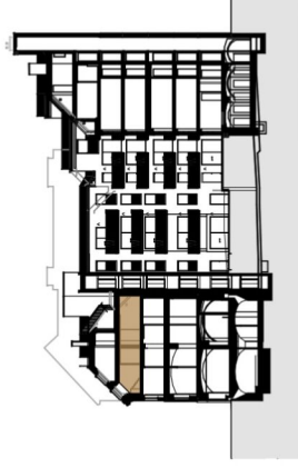
SCHNITT 1-1
