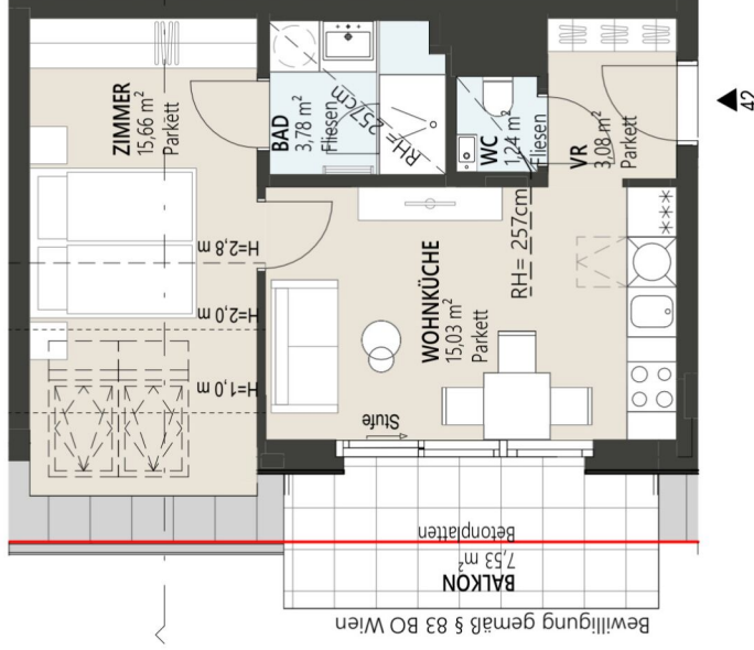
Schnitt schematisch
