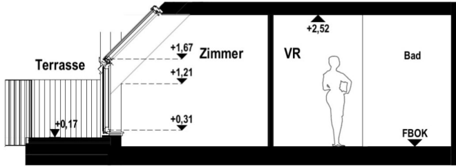
Schnitt
