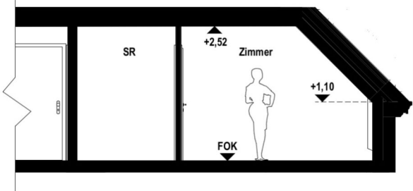
Schnitt
