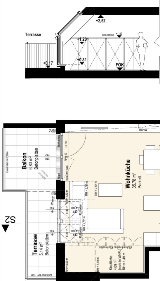
Schnitt 2
