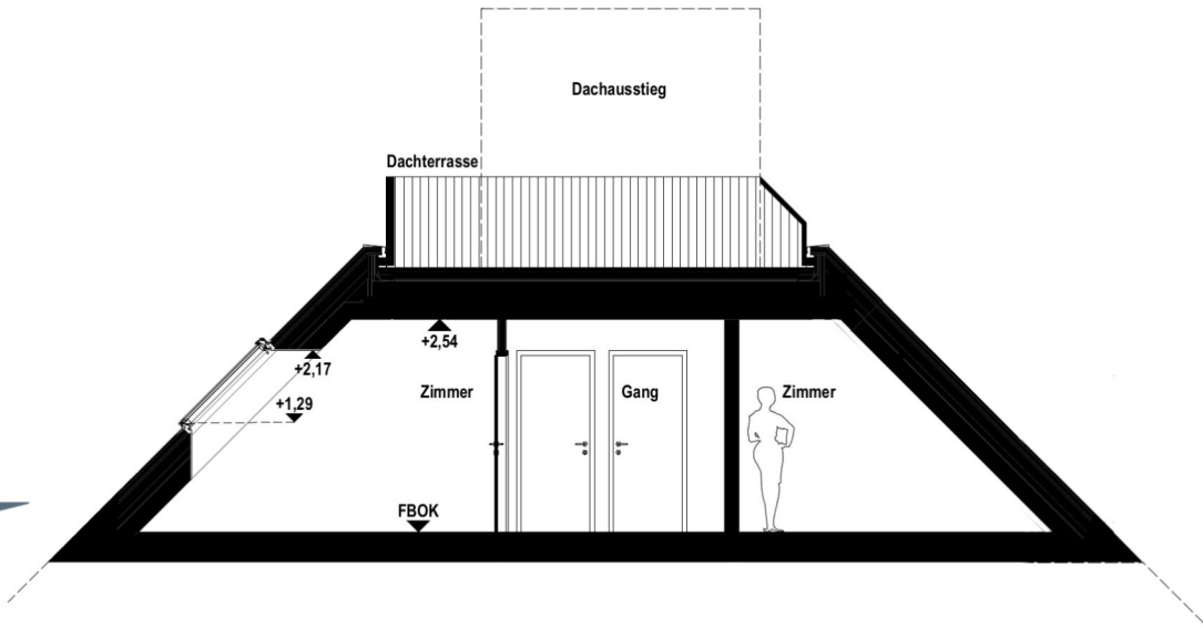
Schnitt
