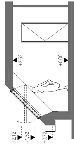
Schnitt 2
