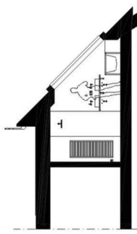
SCHNITT BAD
