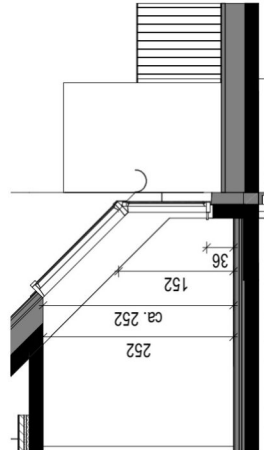
Schnitt 44.A
