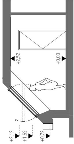
Schnitt 1
