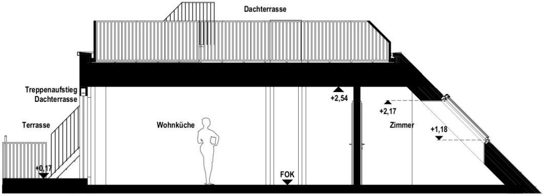
Schnitt
