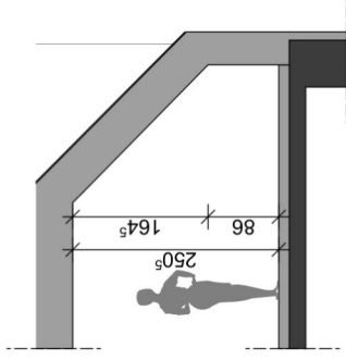
SCHNITT 2-2
