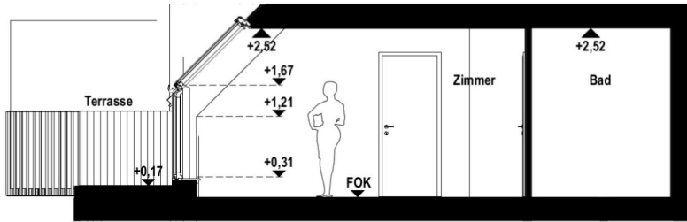
Schnitt
