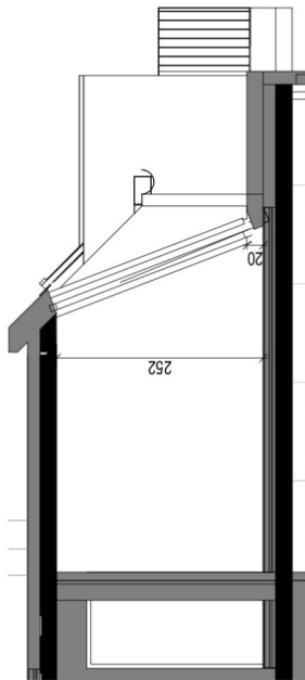
Schnitt 41B
