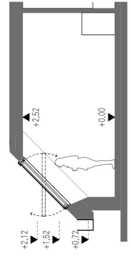
Schnitt 1
