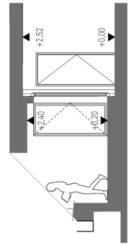
Schnitt 2
