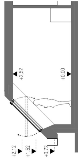
Schnitt 1
