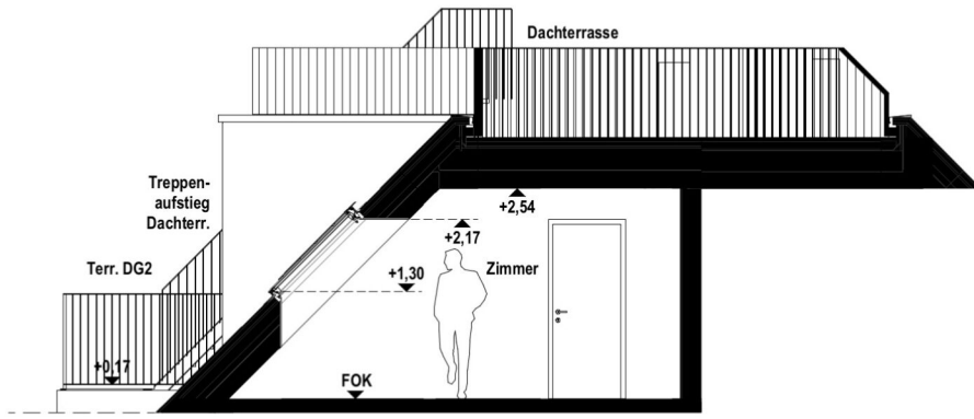
Schnitt
