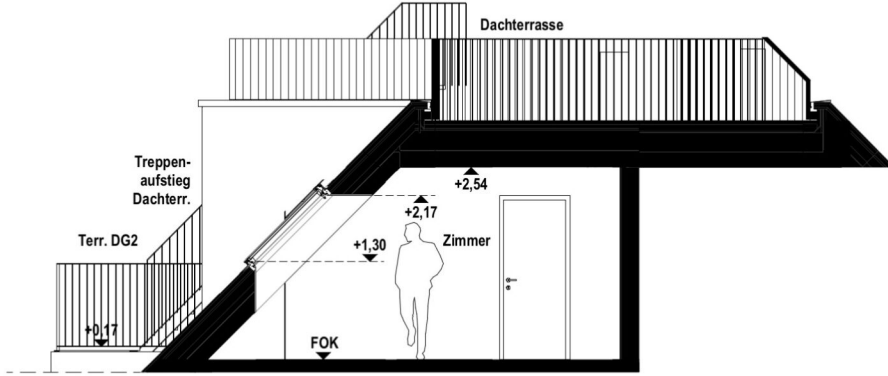
Schnitt
